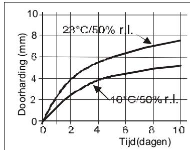
Schema 1: Uithardingsnelheid voor Sikaflex®-521 UV
